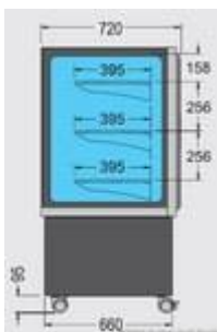
23120005- Seitenskizze
